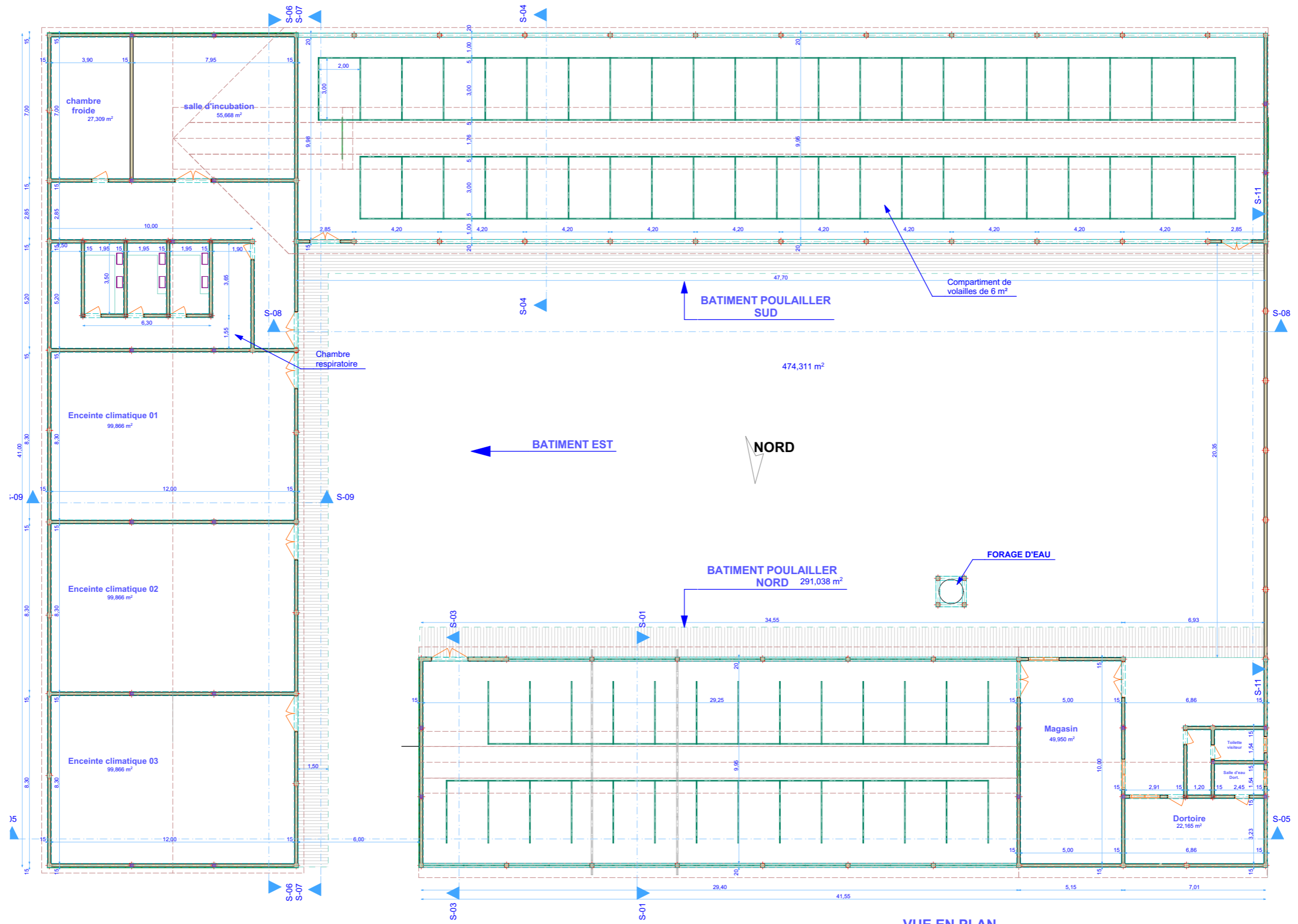
VUE EN PLAN Echl. 1/200
